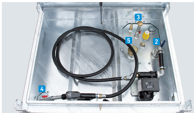
Ausrüstung: Pumpe R50 230, Grenzwertgeber
